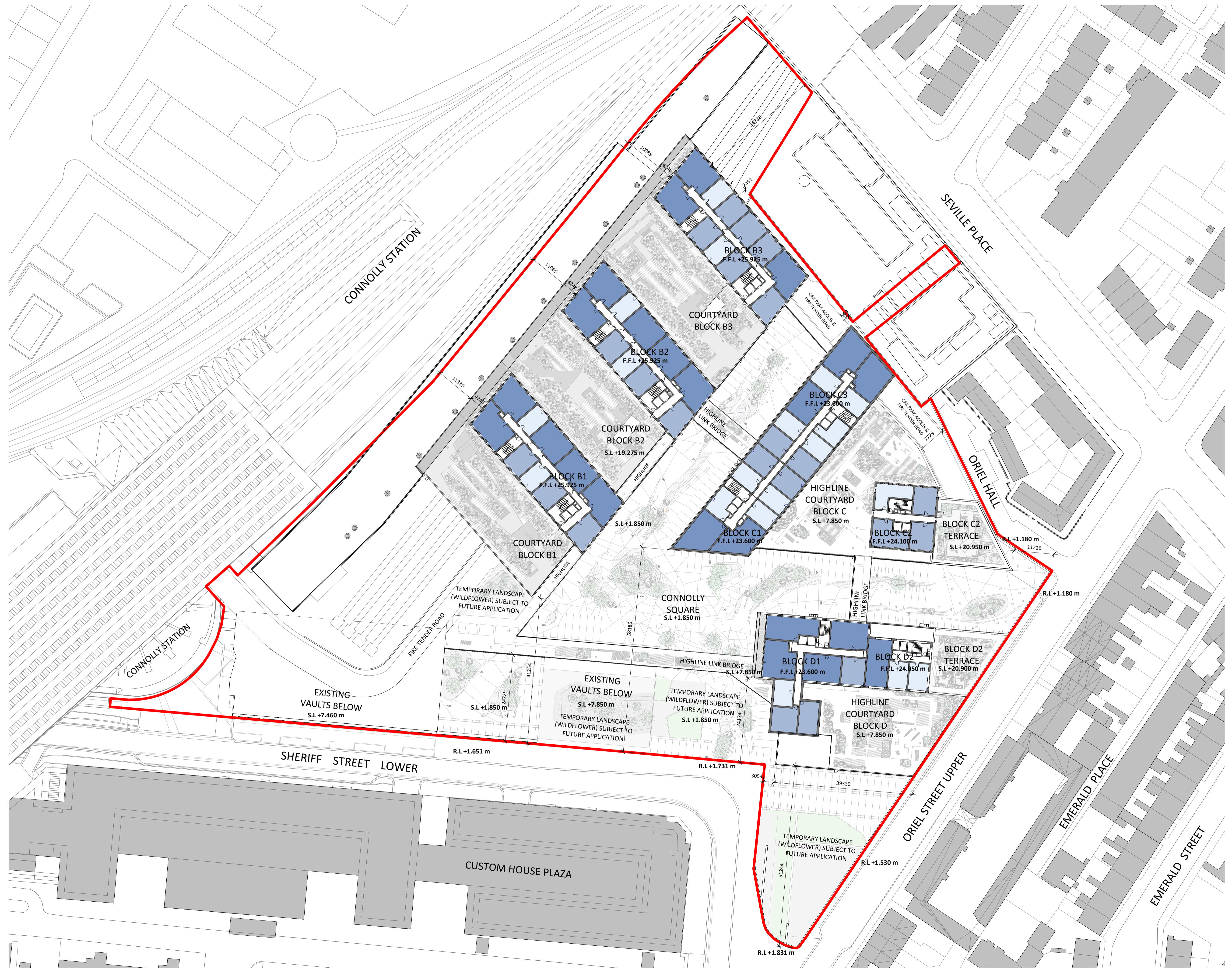
1 SITE LAYOUT PLAN - LEVEL 06 1 : 500
